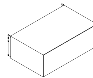
1 Cassetto in legno 1 Wooden drawer H 296 - P 540 L 600 - 900 - 1200
