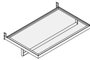
Ripiano in vetro con asta portabiti Glass shelf with clothes rod SP 41 - P 540 W 600 - 900 - 1200 - Custom
