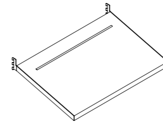
Ripiano in legno per scarpe Wooden shoe shelf SP 41 - P 350 / 540 W 600 - 900 - 1200 - Custom
