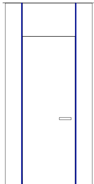
Porta pivot con soprapporta 61mm Pivot door with transom panel 61mm H 1800 / 3200 L 700 / 1500
