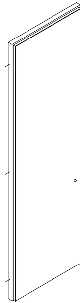
Anta a battente Swing door SP 61 H 1800 / 3200 L 600 / 1200 - Custom
