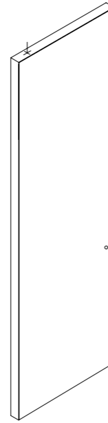
Anta pivot senza battute laterali Pivot door not rebated SP 61 H 1800 / 3200 L 700 / 1500 - Custom
