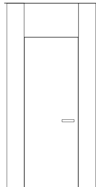
Porta pivot senza battuta con soprapporta 61mm Pivot door without rebated with transom panel 61mm H 1800 / 3200 L 700 / 1500
