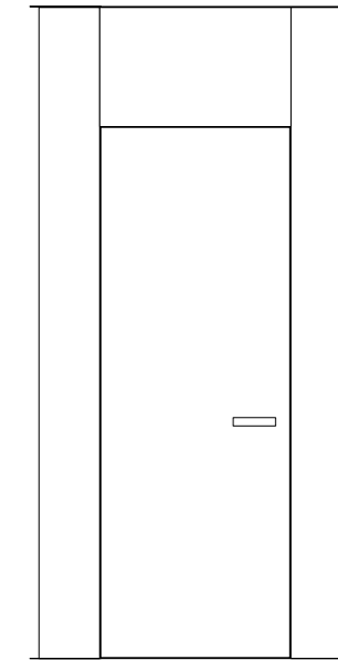
Porta pivot senza battuta con soprapporta 20mm Pivot door without rebated with transom panel 20mm H 1800 / 3200 L 700 / 1500
