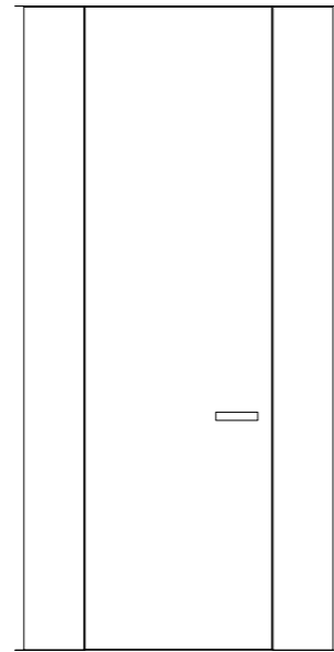
Porta pivot senza battuta a tutta altezza Pivot door without rebated full height H 1800 / 3200 L 700 / 1500
