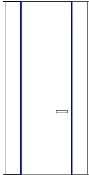
Porta a battente a tutta altezza Swing door full height H 1800 / 3200 L 600 / 1200
