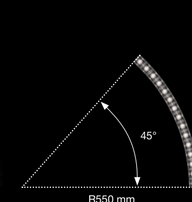
Round module 45° 5,4W - 829 lm
