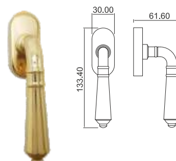
Maniglia per finestra Window handle
