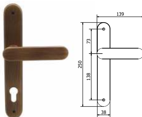
Maniglia su placca Handle on plate
