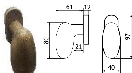
Maniglia per finestra Window handle
