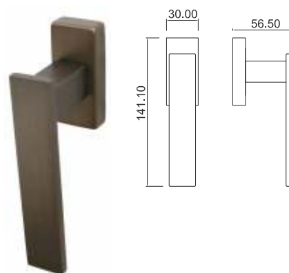
Maniglia per finestra Window handle
