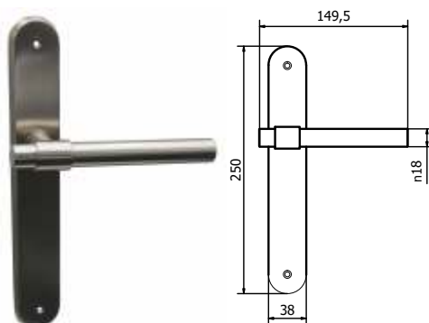
Maniglia su placca Handle on plate
