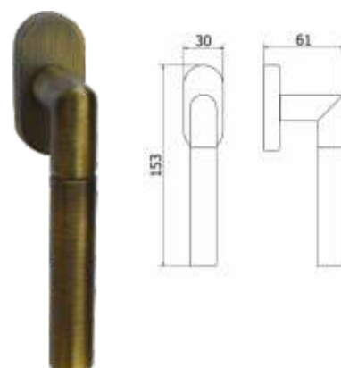
Maniglia per finestra Window handle
