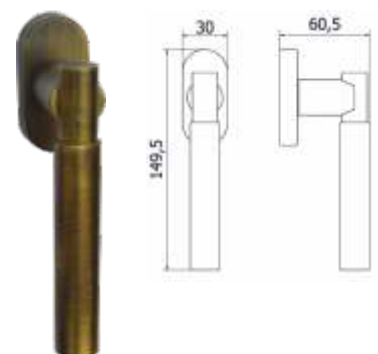
Maniglia per finestra Window handle
