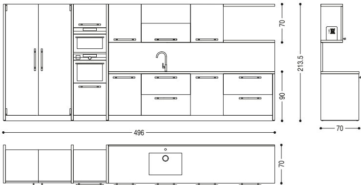
CM: L. 496 · P. 70 · H. 90/213,5
