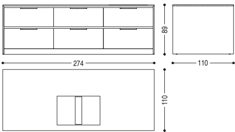
ISOLA - ISLAND - INSEL CM: L. 274 · P. 110 · H. 89
