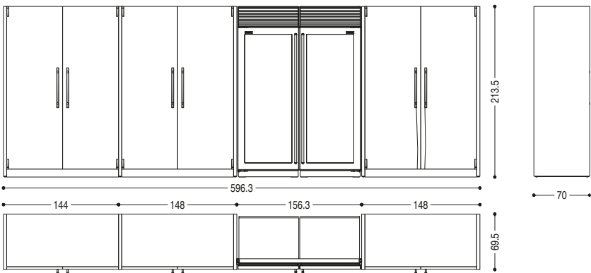
LATO 2 - SIDE 2 - SEITE 2 CM: L. 596,3 · P. 69,5 · H. 213,5
