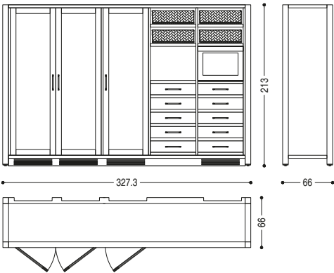
LATO 2 - SIDE 2 - SEITE 2 CM: L. 327,3 · P. 66 · H. 213
