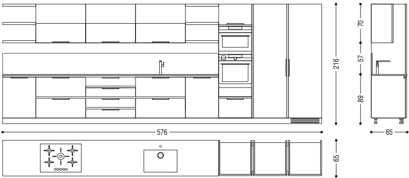
CM: L. 576 · P. 65 · H. 89/216
