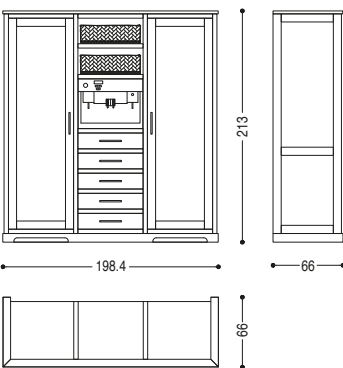
LATO 2 - SIDE 2 - SEITE 2 CM: L. 198,4 · P. 66 · H. 213
