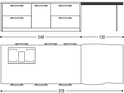
ISOLA - ISLAND - INSEL CM: L. 378 · P. 120 · H. 90
