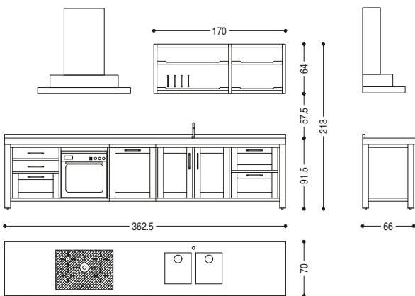
LATO 1 - SIDE 1 - SEITE 1 CM: L. 362,5 · P. 66/70 · H. 91,5/213
