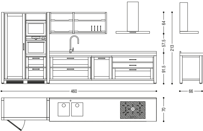
LATO 1 - SIDE 1 - SEITE 1 CM: L. 460 · P. 66/70 · H. 91,5/213
