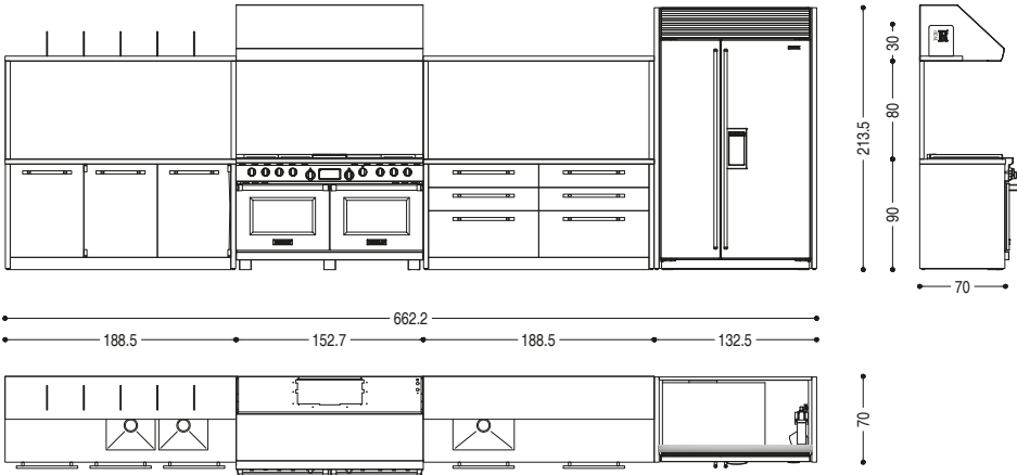
LATO 1 - SIDE 1 - SEITE 1 CM: L. 662,2 · P. 70 · H. 90/213,5
