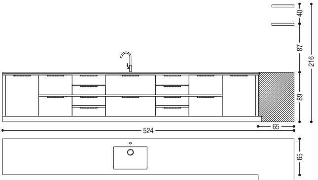
LATO 2 - SIDE 2 - SEITE 2 CM: L. 528 · P. 65 · H. 89/216
